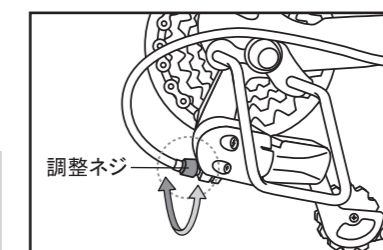
後変速機(リアディレーラー)
